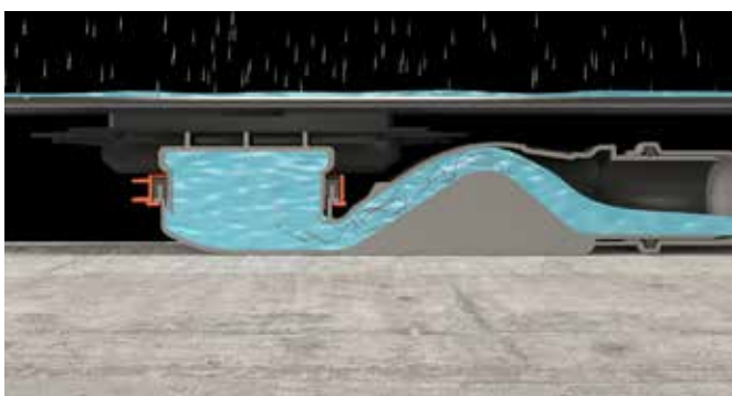
Effetto autopulente grazie all'alta velocità di deflusso
